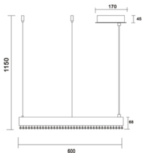
Габаритные размеры
