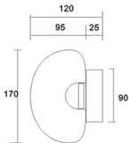
Габаритные размеры
